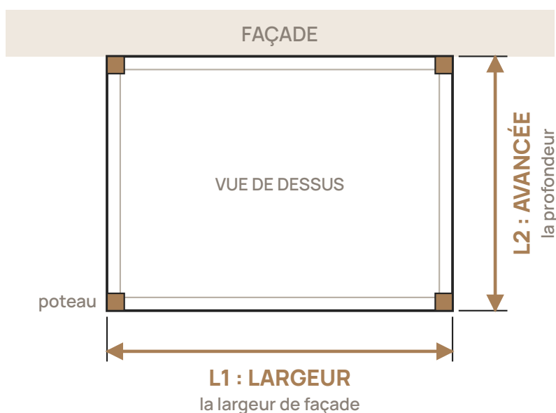
Figure 1 – Vue de dessus : L1, la largeur de façade, et L2, l'avancée. Les deux se prennent hors tout
