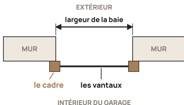
Figure 3 – En applique intérieure : le cadre se fixe contre le mur intérieur du garage, autour de l'ouverture
