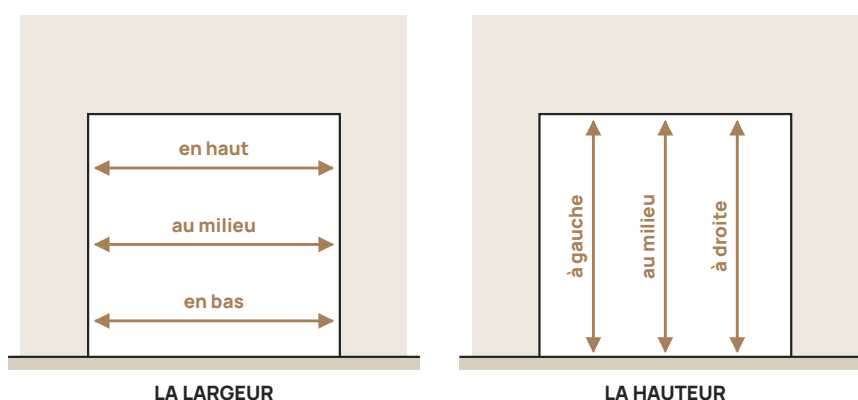
Figure 2 — La largeur et la hauteur de la baie, chacune mesurée en trois points
