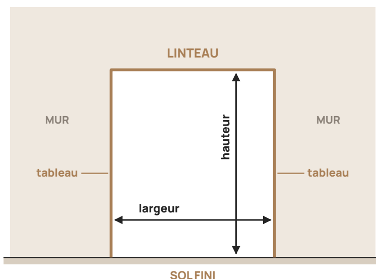
Figure 1 — La baie : sa largeur, d'un tableau à l'autre ; sa hauteur, du sol fini au linteau
