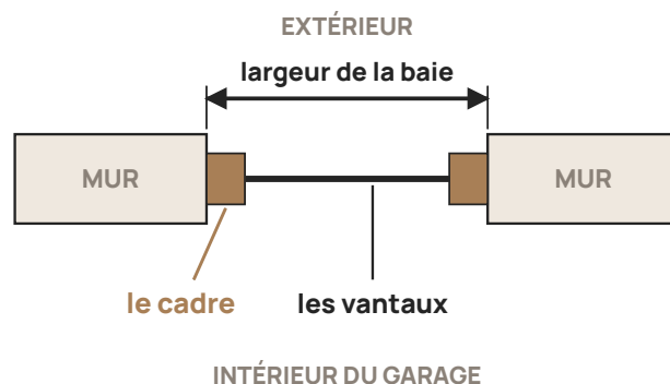
Figure 4 – En tunnel (« entre mur ») : le cadre se loge dans l'épaisseur de l'ouverture
