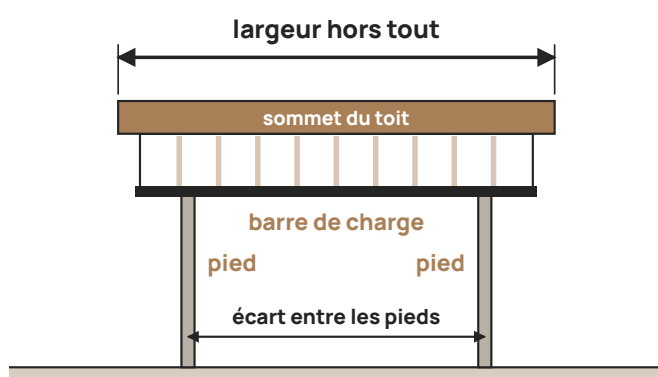
Figure 1 — La largeur hors tout : la largeur totale du store, d'un bout à l'autre. Les pieds sont en retrait
