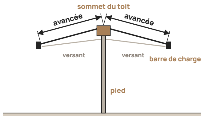
Figure 2 — L'avancée par côté : du sommet du toit à la barre de charge, la même sur les deux versants
