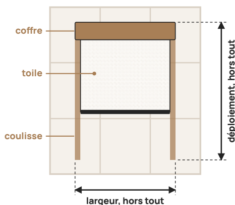
Figure 1 — Le store vu à plat, toile à moitié sortie : la largeur et le déploiement se prennent hors tout
