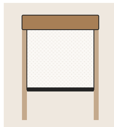
Figure 4 – Coulisses latérales : la toile coulisse dans deux profils latéraux qui la recouvrent
