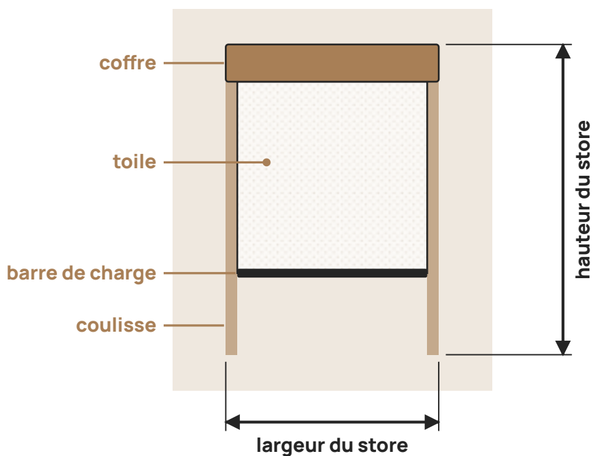
Figure 1 – Le store vu de face : sa largeur et sa hauteur
