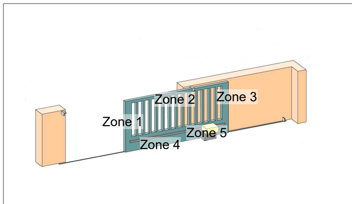
Illustratie 1: Veiligheidsafstand
