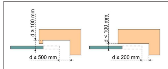
Abbildungen 1: Sicherheitsabstand
