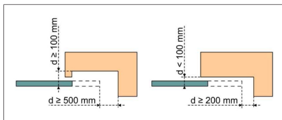
Obrázek 1: Bezpečnostní vzdálenost
