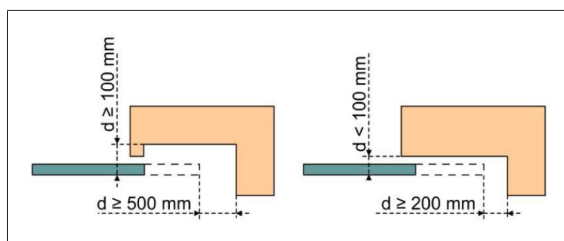
Illustratie 1: Veiligheidsafstand
