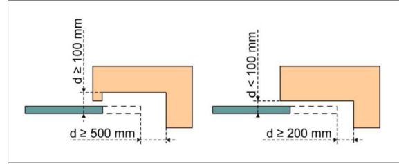
Şekil 1: Güvenlik mesafesi
