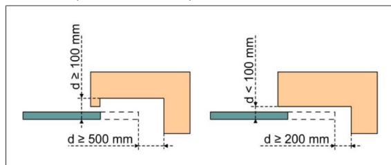
Εικόνα 1: Απόσταση ασφαλείας
