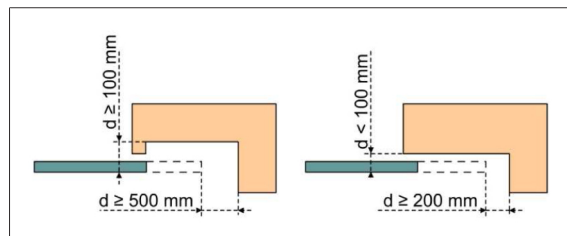
Ábra 1: Biztonsági távolság
