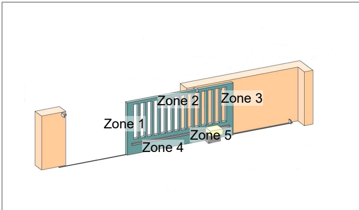
Abbildungen 1: Sicherheitsabstand
