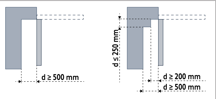
Ilustración 1: Distancias de seguridad Obturación deformable que garantiza una distancia de seguridad de 25 mm en posición comprimida
