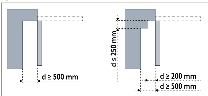
Obrázek 1: Bezpečnostní vzdálenosti
