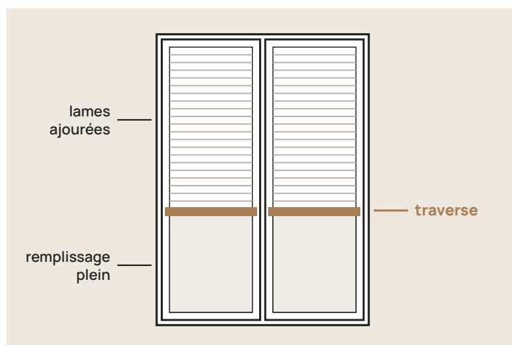
Figure 3 — Volet mixte : lames ajourées en haut, remplissage plein en bas, séparés par une traverse
