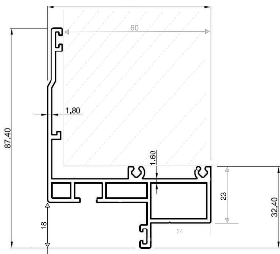
Figure 4 – Le précadre aluminium : coupe cotée, en millimètres
