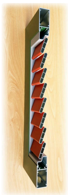
Figure 1 — Vantail à lames ajourées américaines , en coupe : le cadre et ses lames
