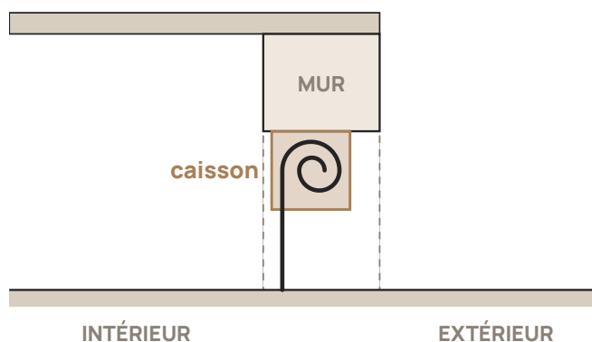
Figure 5 – Entre murs, enroulement extérieur : le caisson se loge entre les murs, le tablier s'enroule côté extérieur
