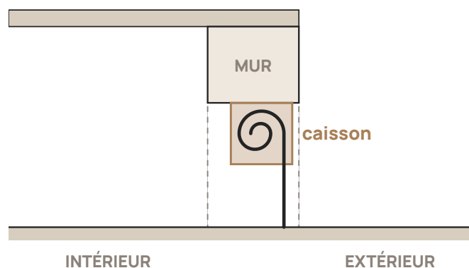
Figure 4 – Entre murs, enroulement intérieur : le caisson se loge entre les murs de l'ouverture, le tablier s'enroule côté intérieur
