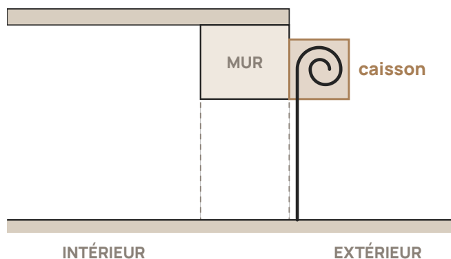
Figure 3 – Applique extérieure : le caisson est fixé à l'extérieur du bâtiment
