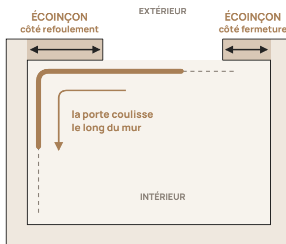
vue de dessus · ici, refoulement à gauche
