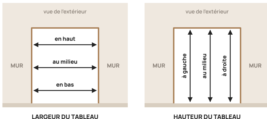
Figure 1 – Le tableau vu de l'extérieur : sa largeur et sa hauteur, chacune mesurée en trois points
