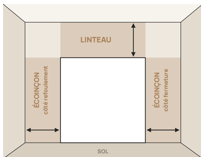
vue de l'intérieur du garage · ici, refoulement à gauche
