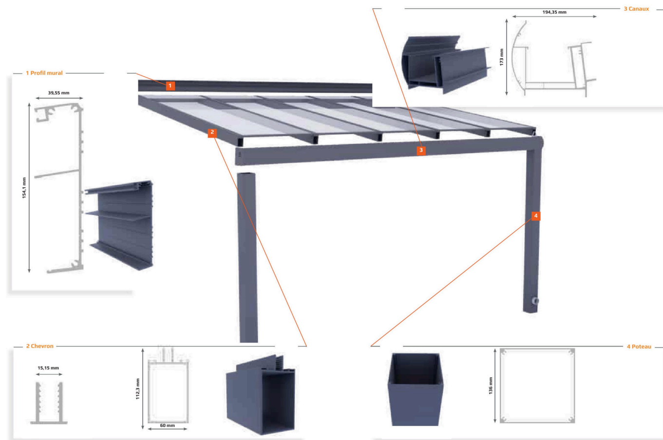
Figure 1 — La pergola en vue éclatée : 1 le profil mural, 2 un chevron, 3 le chéneau, 4 un poteau. Chaque encadré est repris en grand à la page suivante
