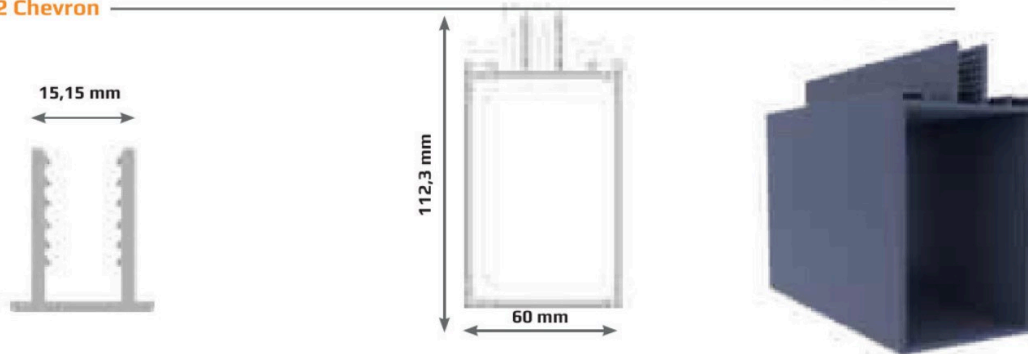
Figure 3 – Repère 2 : le chevron
