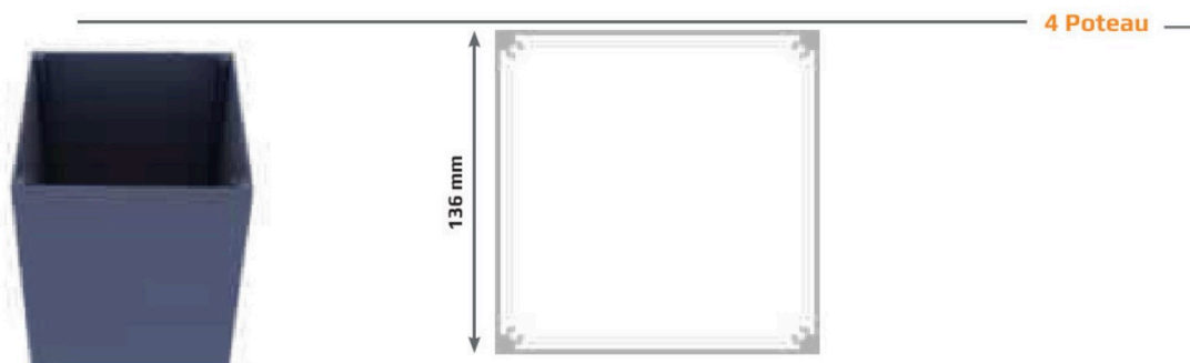
Figure 5 — Repère 4 : le poteau
