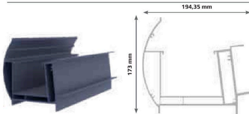
Figure 4 – Repère 3 : le chéneau
