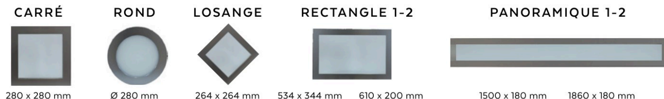
Figure 11 – Les hublots à cadre Alunox
