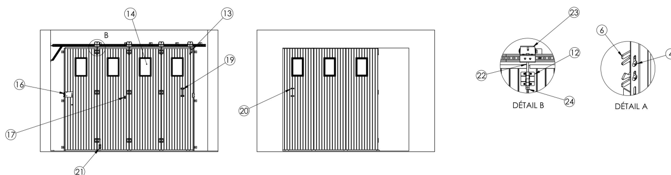
Figure 1 – À gauche, la porte vue de l'intérieur du garage ; au centre, vue de l'extérieur ; à droite, le détail B (un chariot, boulonné sur une charnière du haut) et le détail A (la butée d'arrêt de la serrure)
