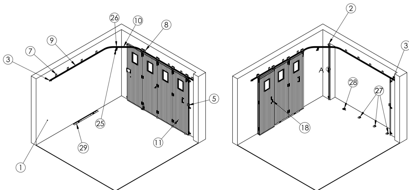
Figure 2 – L'intérieur du garage : à gauche la porte fermée, à droite la porte ouverte, rangée le long du mur de refoulement
