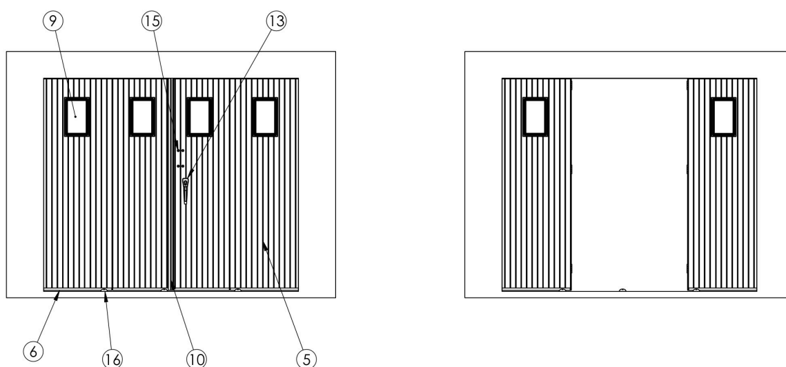
Figure 1 – La porte vue de face : fermée (à gauche) et ouverte (à droite)
