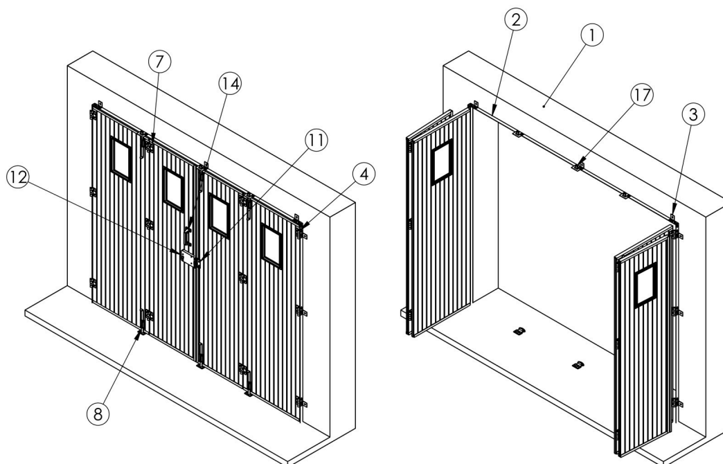
Figure 2 – L'intérieur du garage : à gauche la porte fermée, à droite la porte ouverte, les vantaux repliés de chaque côté
