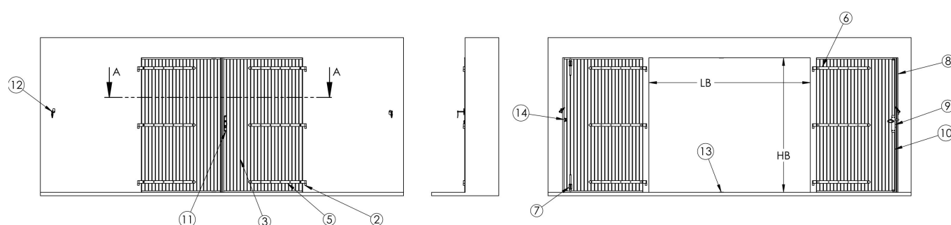
Figure 1 – À gauche, la porte fermée vue de l'extérieur, puis son profil ; à droite, la porte ouverte : LB est la largeur de la baie, HB sa hauteur
