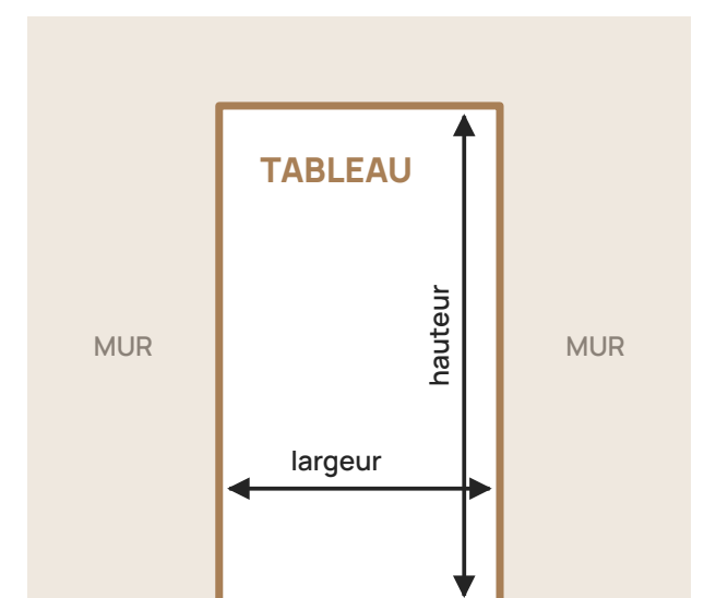
Figure 1 — Le tableau : l'ouverture dans le mur
