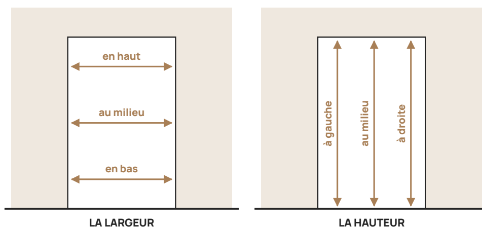
Figure 4 – La largeur et la hauteur de l'ouverture, chacune mesurée en trois points
