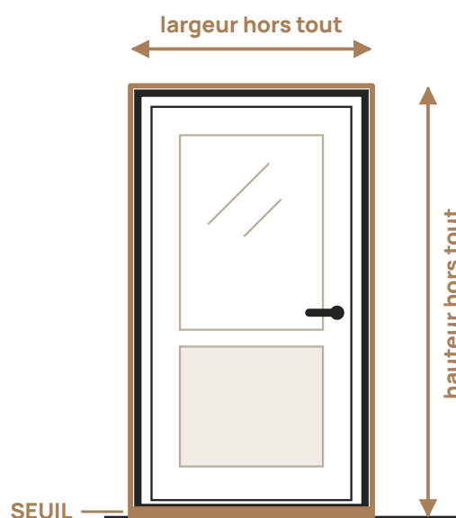
Figure 2 — Le cadre : la porte hors tout, seuil compris
