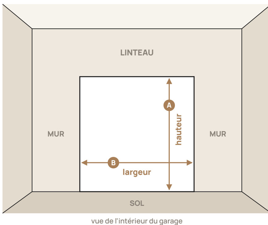
Figure 1 — La baie vue de l'intérieur : A, sa hauteur, du sol au linteau ; B, sa largeur, entre les murs
