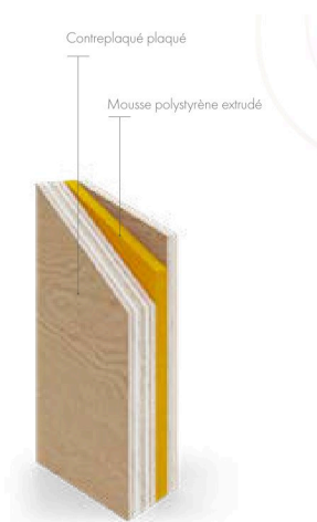
Figure 1 — Le panneau en coupe : les faces en contreplaqué plaqué, la mousse isolante au cœur.
