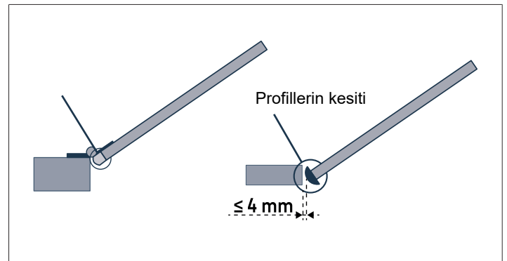
Şekil 2: Mekanik koruma
