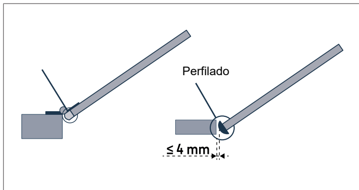
Ilustração 2: Proteção mecânica
