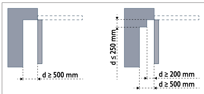
Illustratie 1: Veiligheidsafstanden
