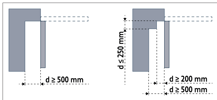
Abbildungen 1: Sicherheitsabstände
