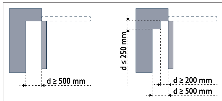
Εικόνα 1: Αποστάσεις ασφαλείας
