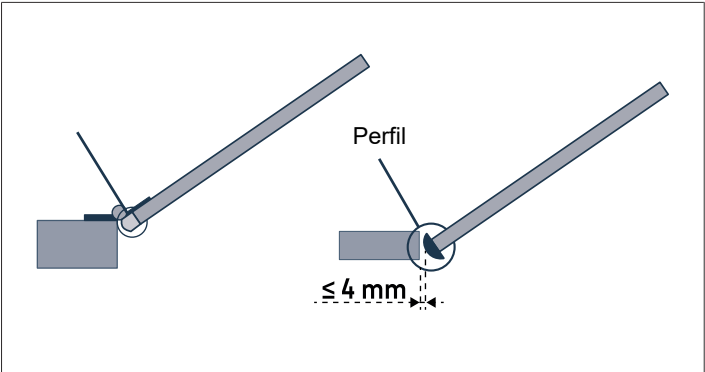
Ilustración 2: Protección mecánica
