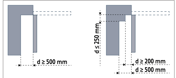
Şekil 1: güvenlik mesafeleri
