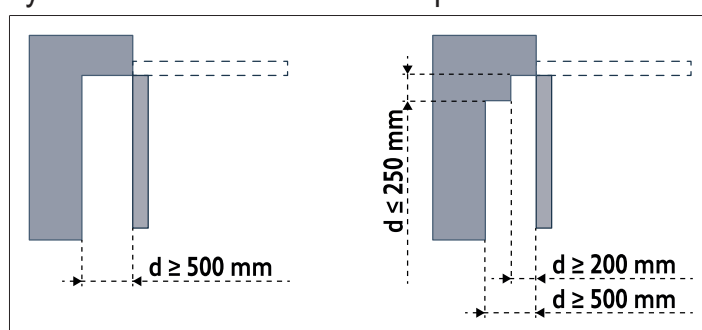
Obrázek 1: Bezpečnostní vzdálenosti
